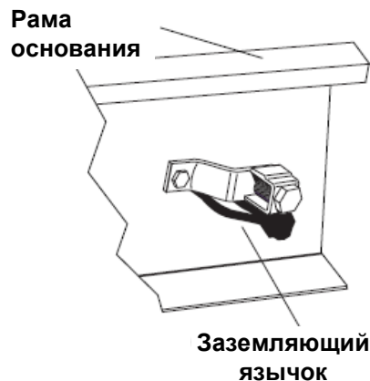
Рисунок 2.2. Заземляющий язычок генератора (типовой)
