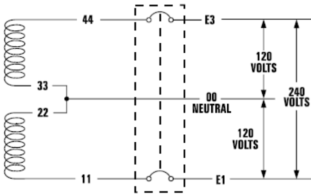
Рисунок 1.2. Статор 4 вывода, 1 фаза
